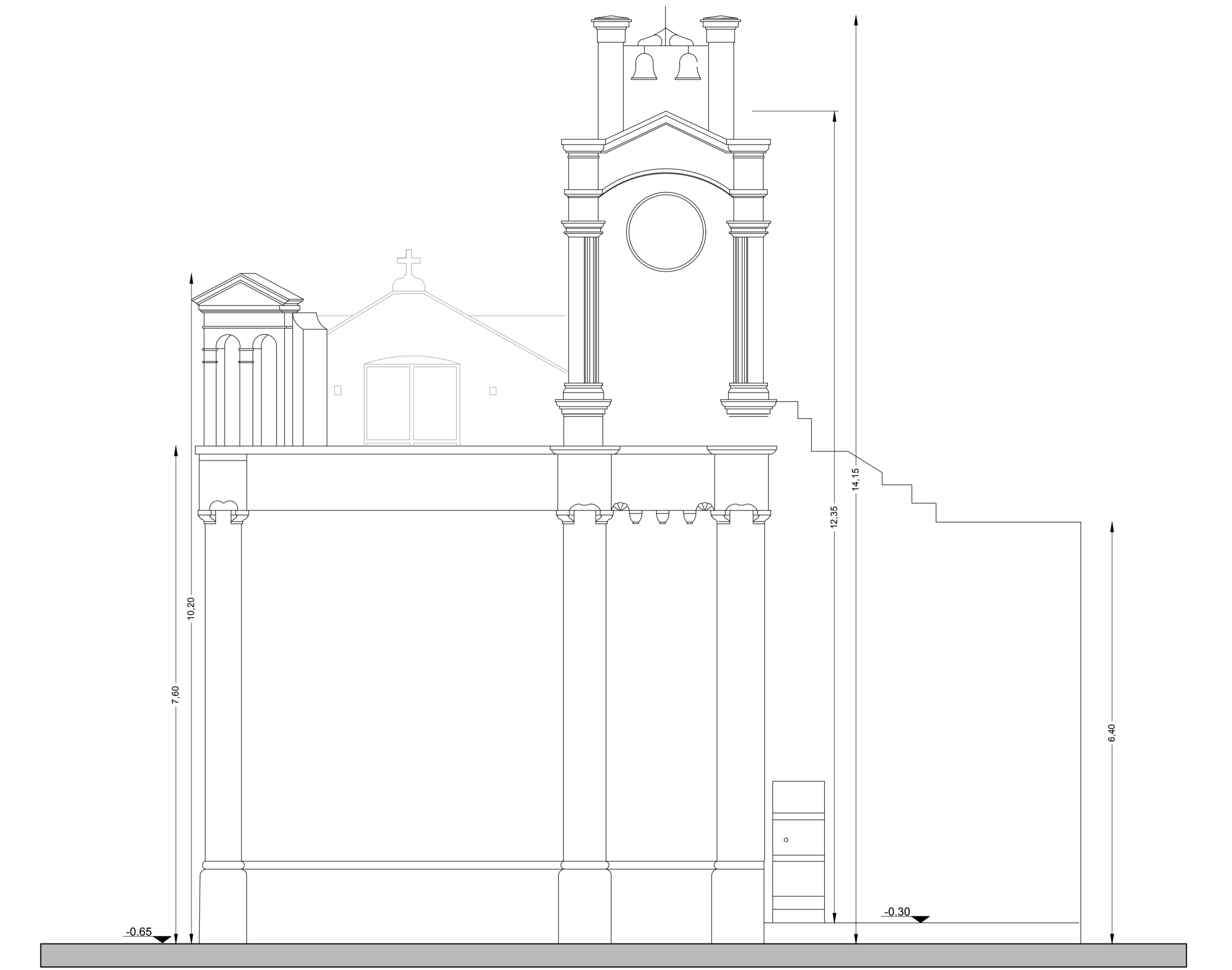
PROSPETTO SU VIA MARCHESE BERNARDINI
