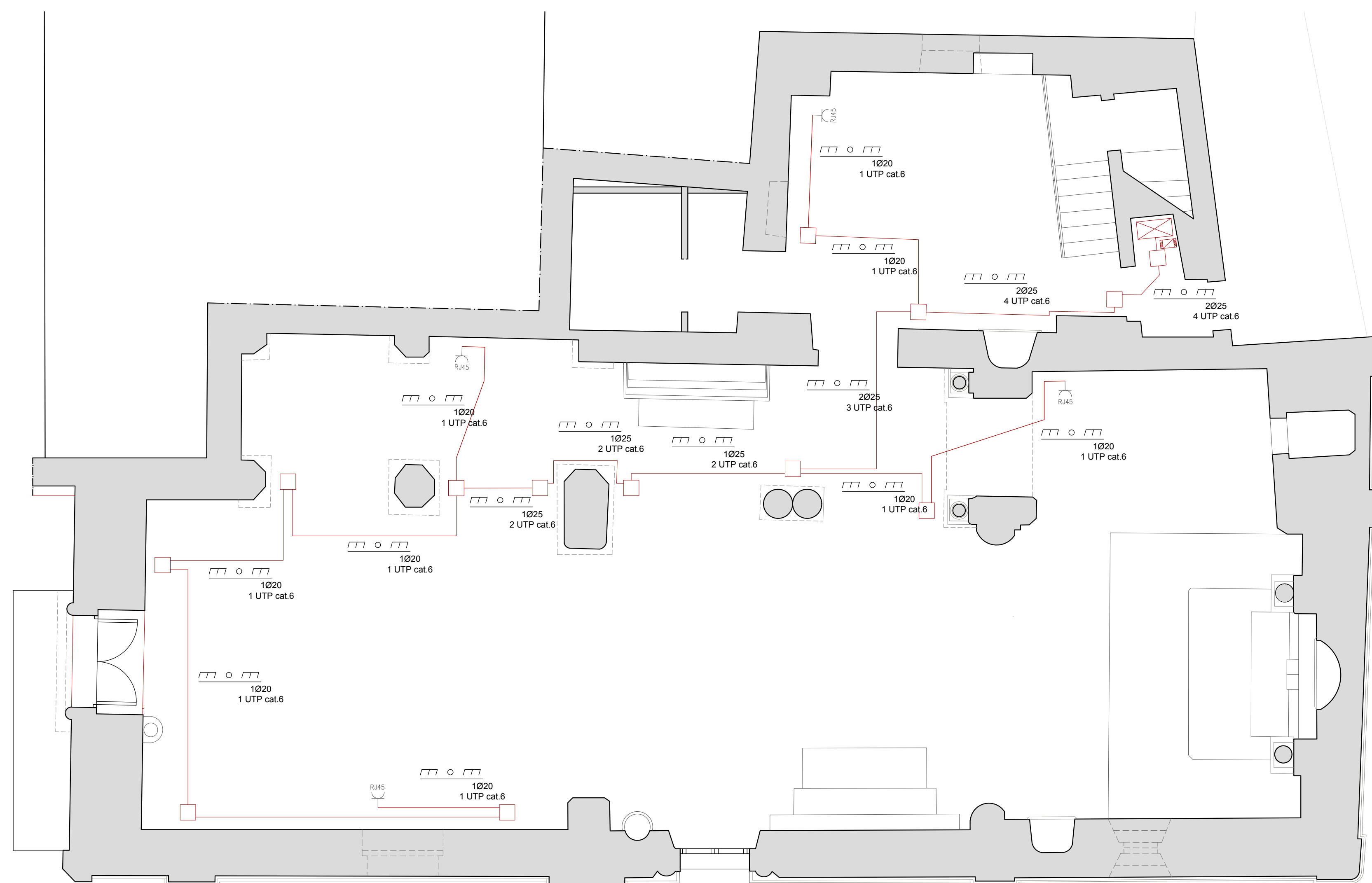
Pianta piano terra - impianto servizi RETE TRASMISSIONE DATI
