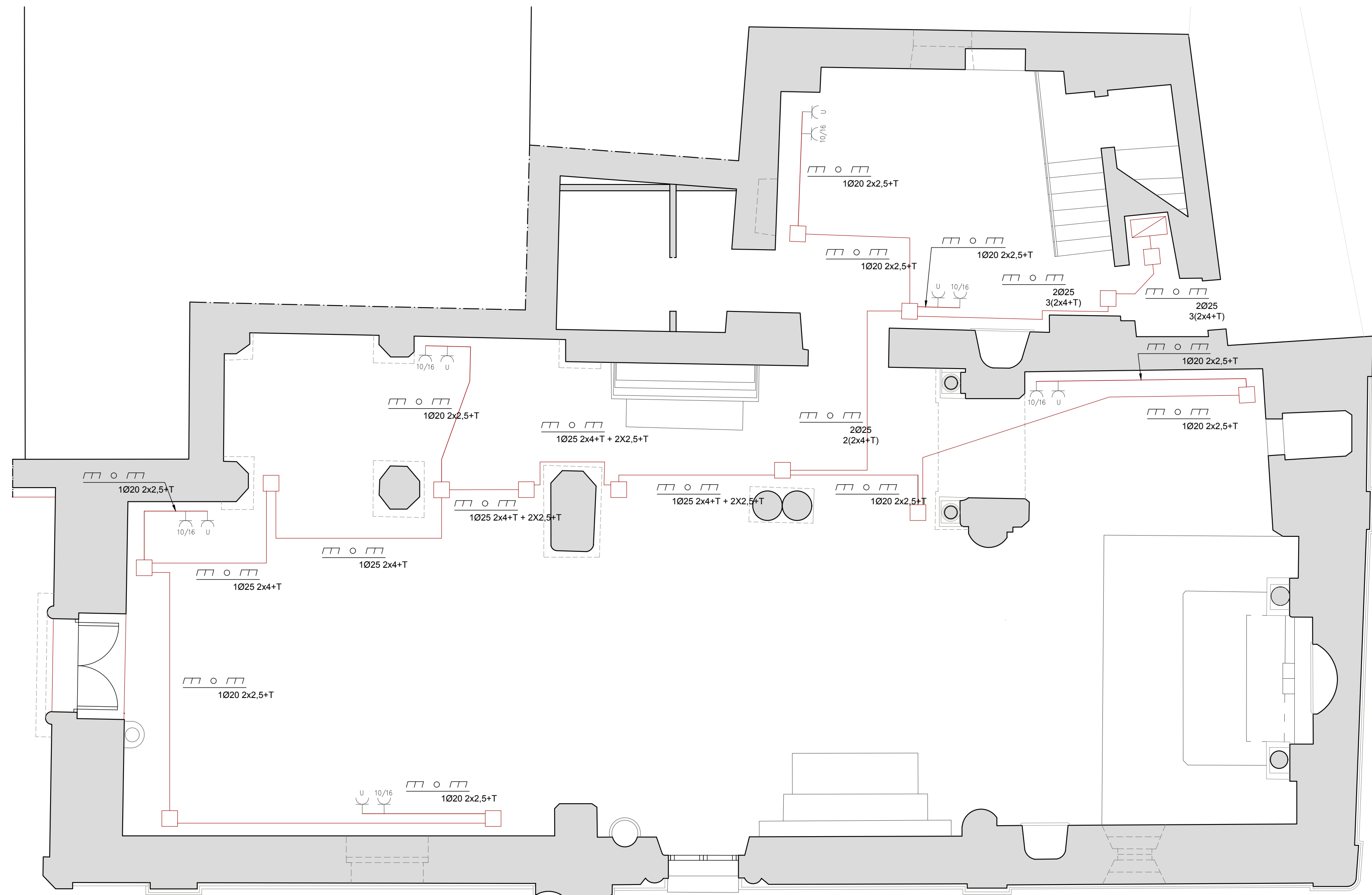
Pianta piano terra - impianto elettrico CIRCUITO PRESE
